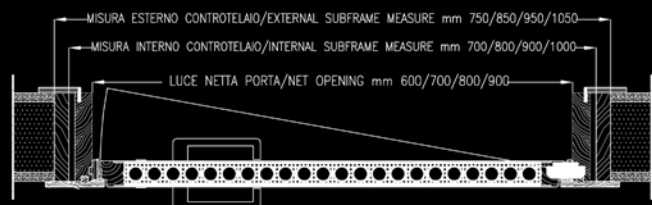
SEZIONE ORIZZONTALE/HORIZONTAL SECTION
